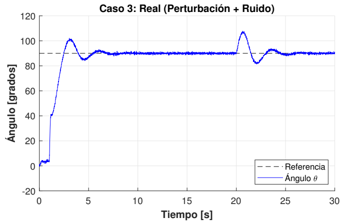
Figura 7. Caso 3 – Ruido: respuesta angular del péndulo con ruido de medición activo. El controlador mantiene la posición estable en torno a la referencia.
